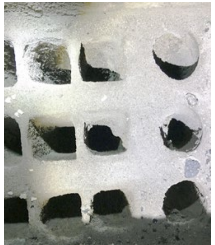
De värmeupptagande ytorna i pannan ses på fotot och för varje millimeter sot ökar rökgastemperaturen med cirka 50 grader. Uppskattningsvis var det cirka 10 millimeter sot på den del som syns på bilden.
